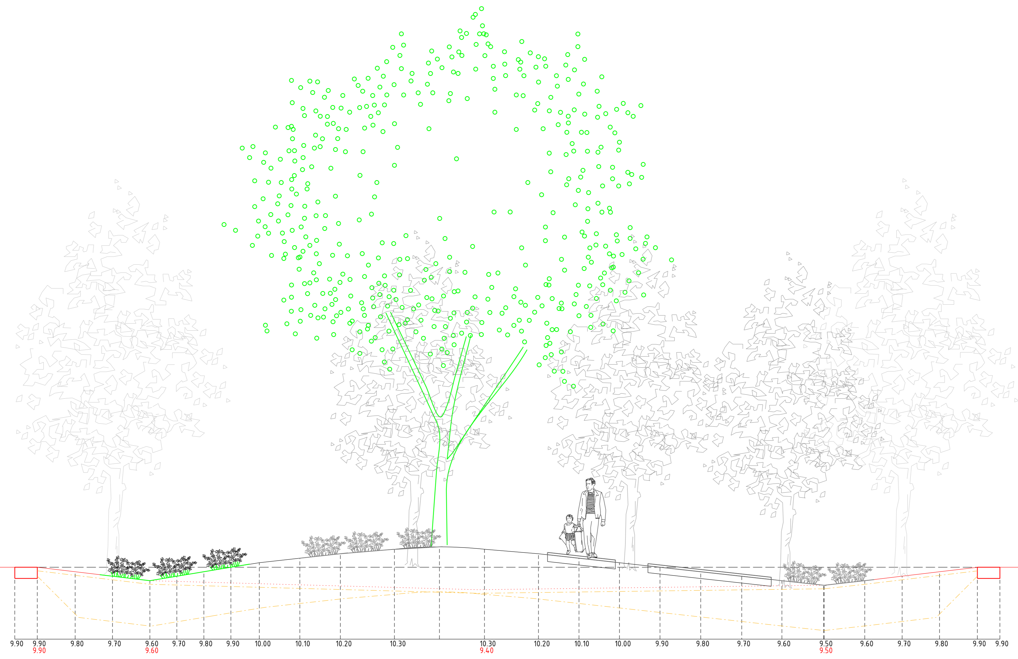
Dwarsprofiel B-B Schaal 1 : 50
