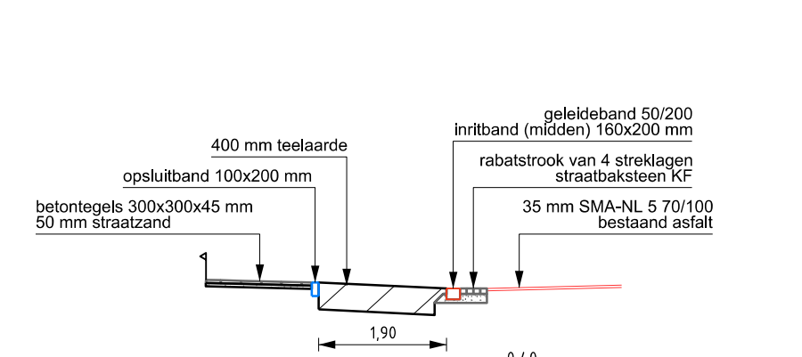
PRINCIPLEDETAIL ter plaatse van plantvakken aan zijzijde van de straat schaal 1:100
