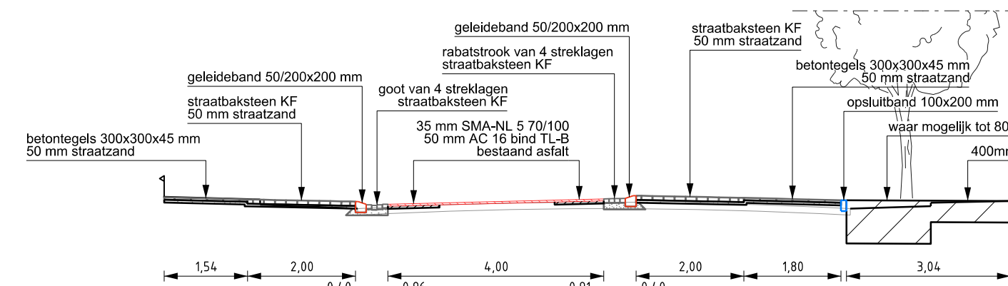
PROFIEL A - A schaal 1:100
