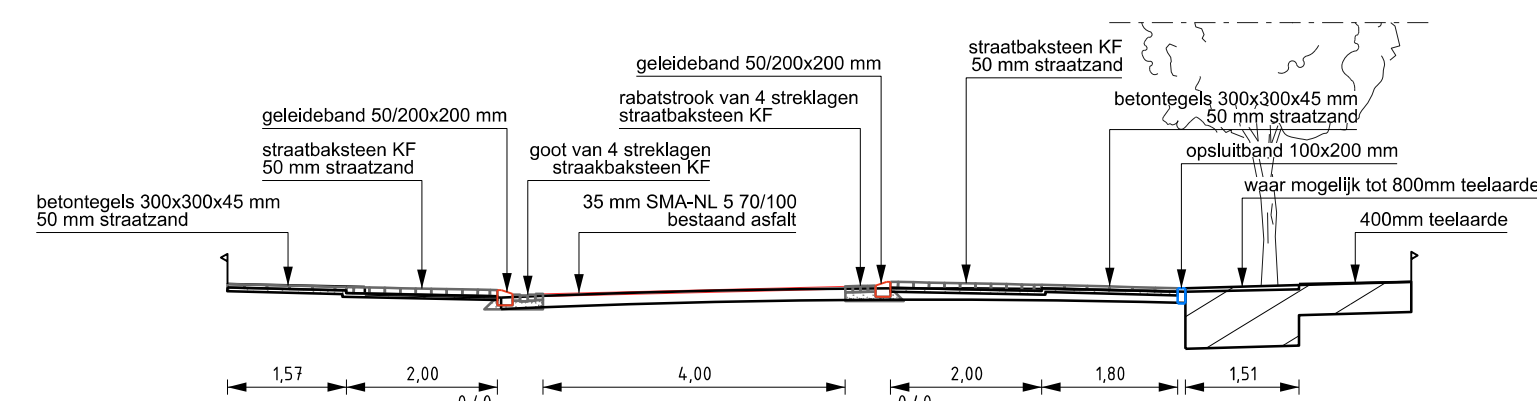
PROFIEL B - B schaal 1:100
