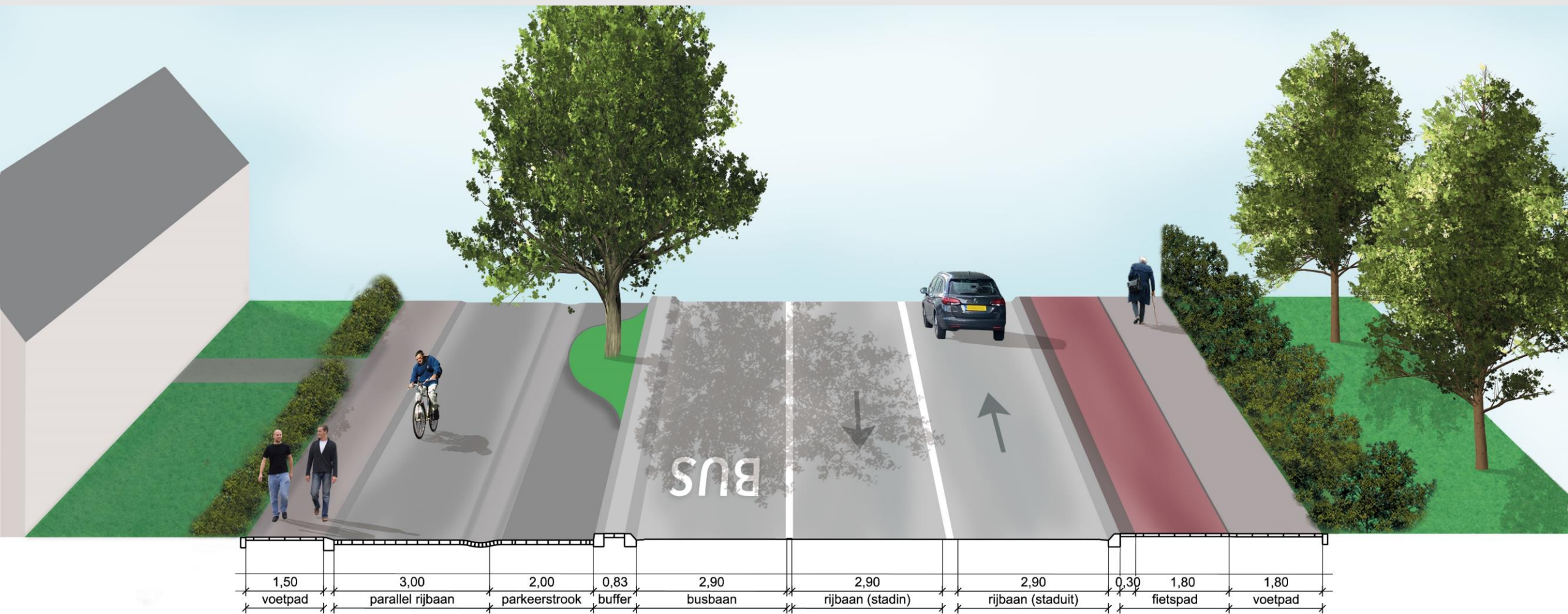
Dwarsprofiel A-A
