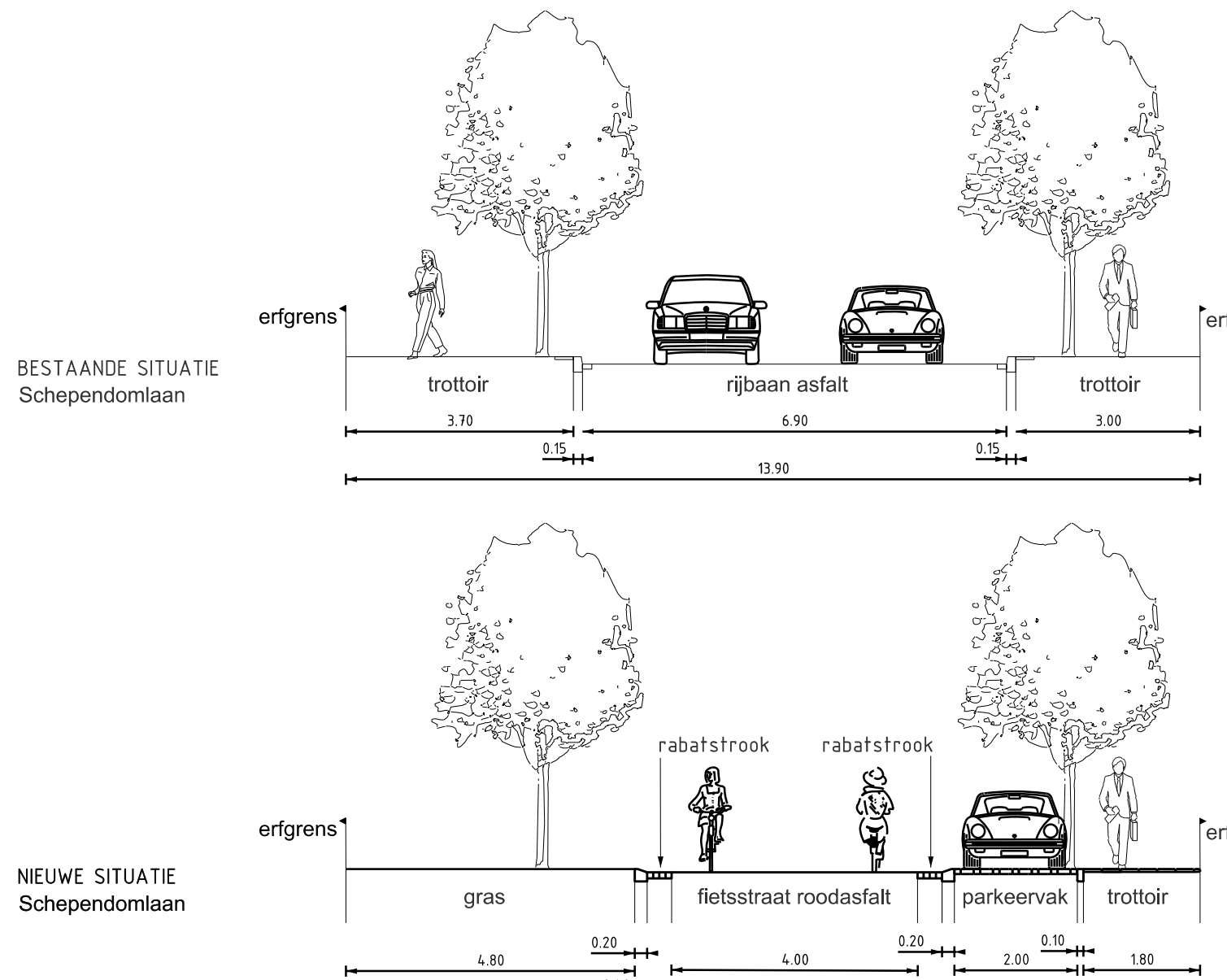
DWARSPROFIEL C-C
