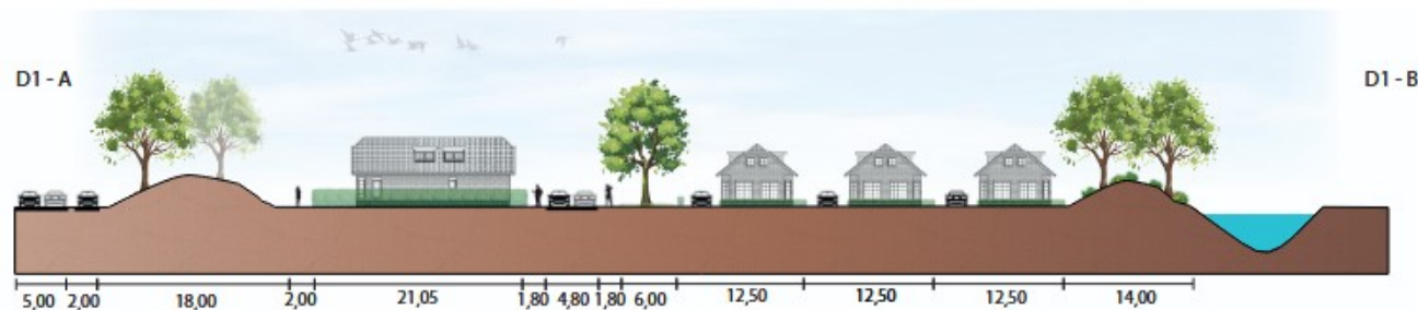
Doorsneden 1:200
