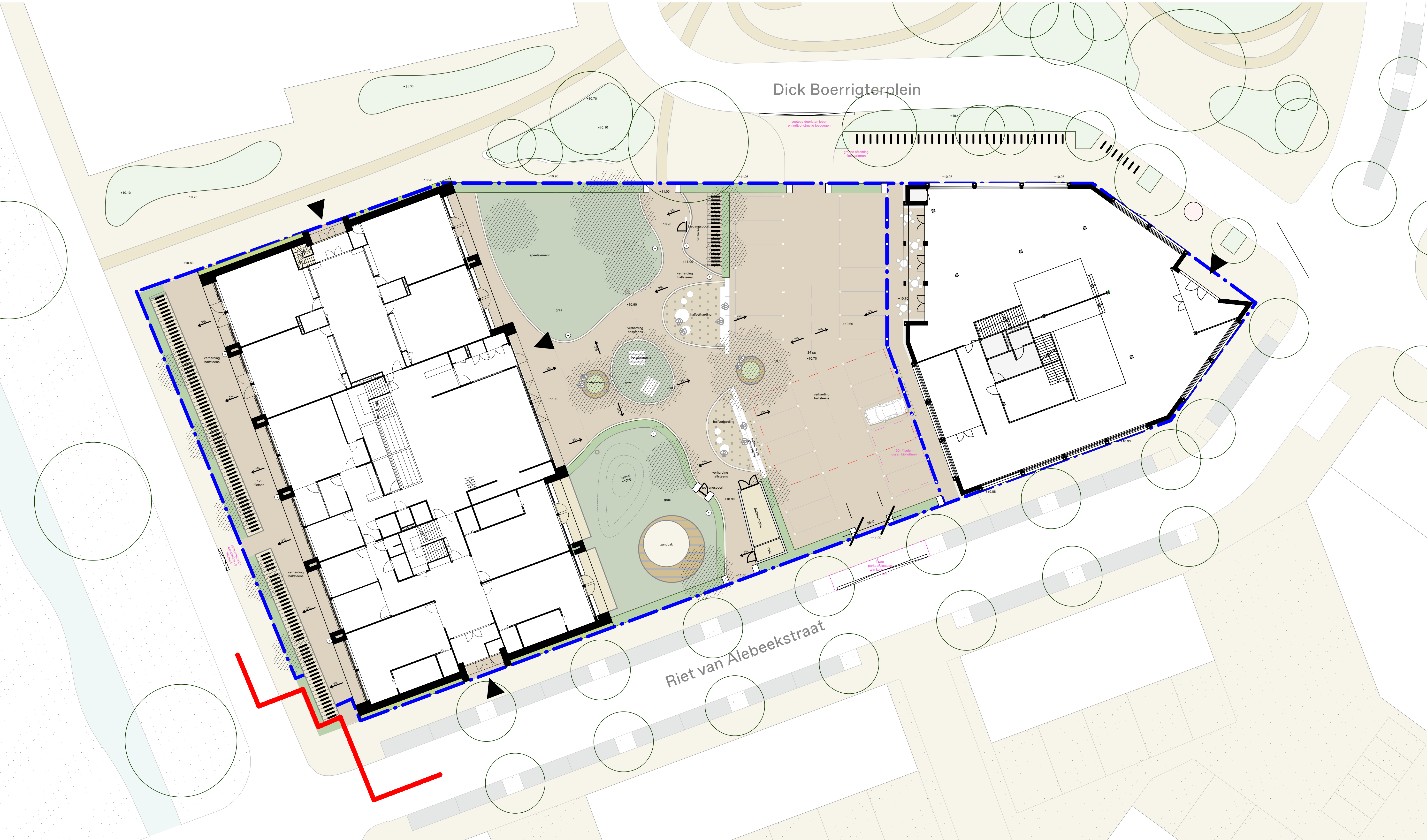
Begane grond Hof van Holland op locatie
